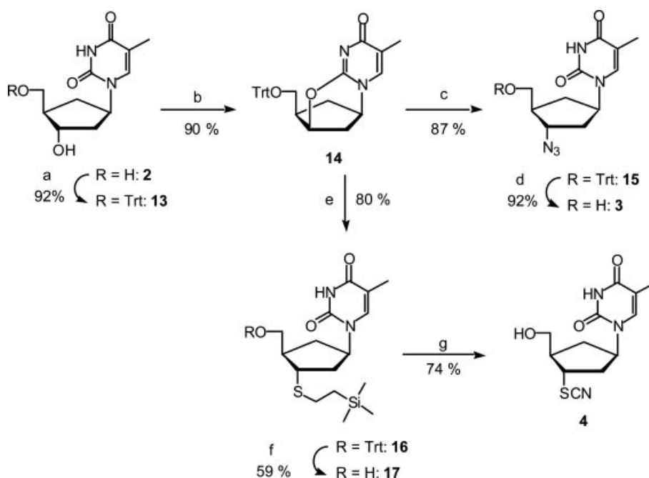
Scheme 1. (a) TrtCl, pyridine, 90 °C, 3 h (b) P(Ph) 3 , DIAD, MeCN, 0 °C, 12 h (c) NaN 3 , DMF, 140 °C, 12 h, (d) TFA, CH 2 Cl 2 /MeOH, room temp., 10 h, (e) 2-(trimethylsilyl)ethanethiol, NaH, DMF, 90 °C, 2 h (f) HCOOH, Et 2 O, room temp. 12 h (g) BrCN, MeOH, room temp. 18 h.
